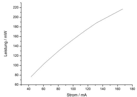
Abbildung 9: Strom-Leistungskurve
