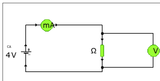
Abbildung 8: Darstellung zum Messen von Spannung und Strom in der Schaltung des Rüttlers
