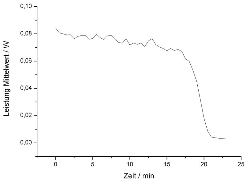
Abbildung 20: Gemittelte Messungen im Leistungs-Zeit Diagramm beim Rütteln mit 35 Hz
