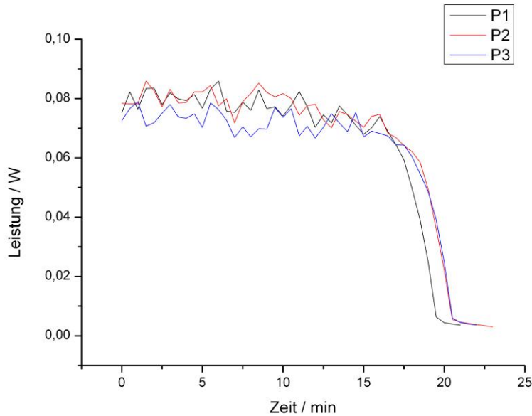
Abbildung 17: Drei Messungen im Leistungs-Zeit Diagramm beim Rütteln mit 15Hz
