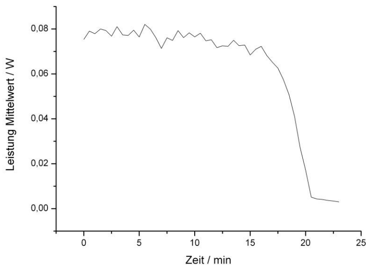
Abbildung 18: Gemittelte Messungen im Leistungs-Zeit Diagramm beim Rütteln mit 15Hz
