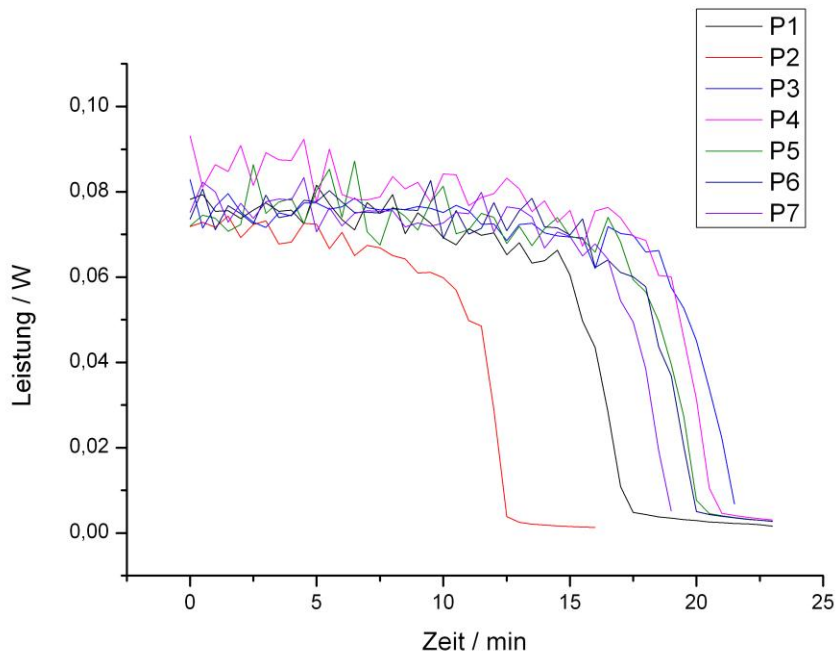
Abbildung 13: Sechs Messungen mit Mittelwertbildung über einer halben Minute
