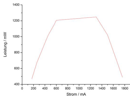
Abbildung 10: Strom-Leistungskurve
