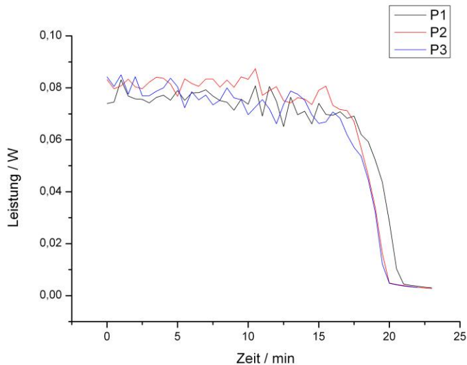
Abbildung 15: Drei Messungen im Leistungs-Zeit Diagramm beim Rütteln mit 5Hz
