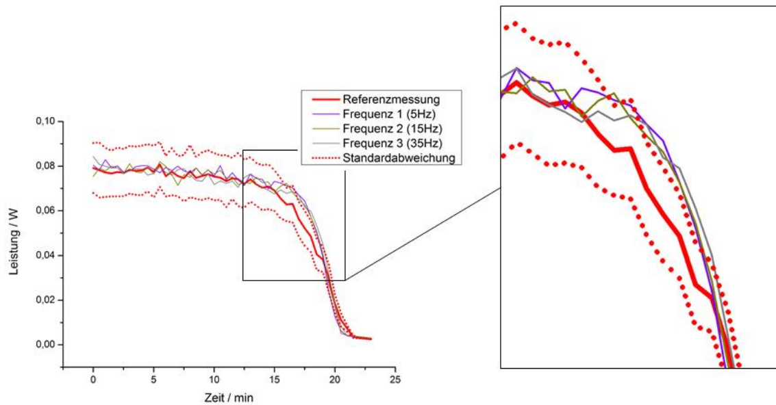
Abbildung 23: gemittelte Referenzmessung mit Standardabweichung und die gemittelte Messung mit anderen Frequenzen
