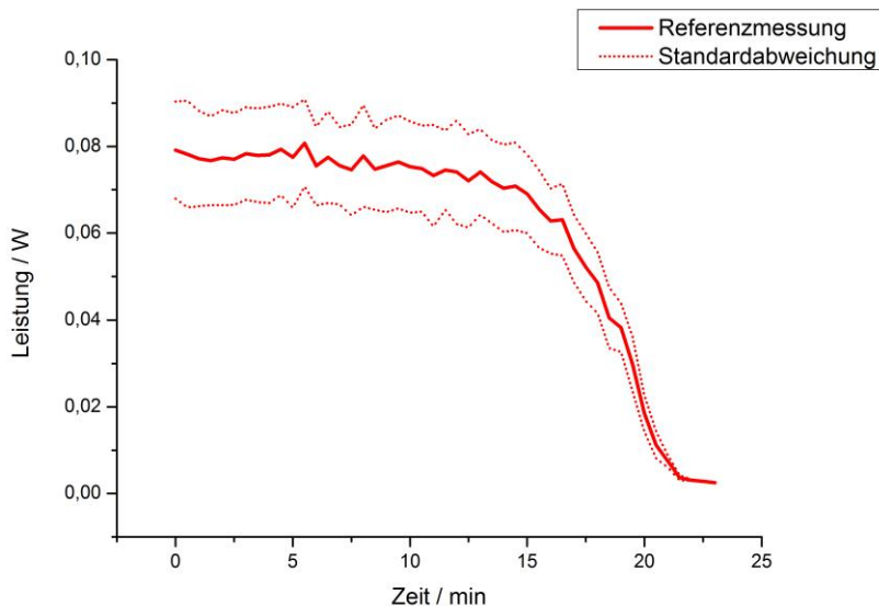
Abbildung 22: Referenzmessung mit Standardabweichung
