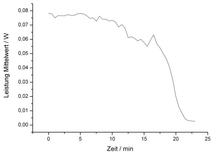
Abbildung 14 Gemittelte Messungen im Leistungs-Zeit Diagramm bei Normalbedingungen
