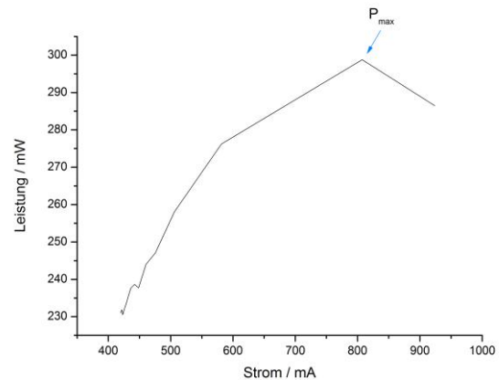
Abbildung 11: : Strom-Leistungskurve
