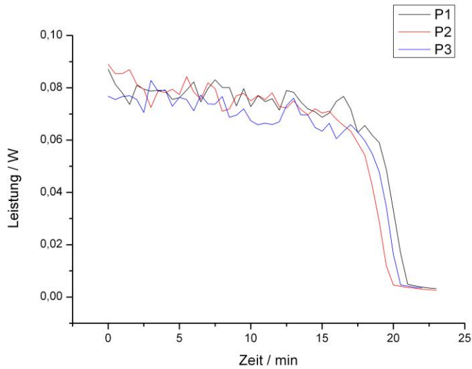
Abbildung 19: Drei Messungen im Leistungs-Zeit Diagramm beim Rütteln mit 35Hz
