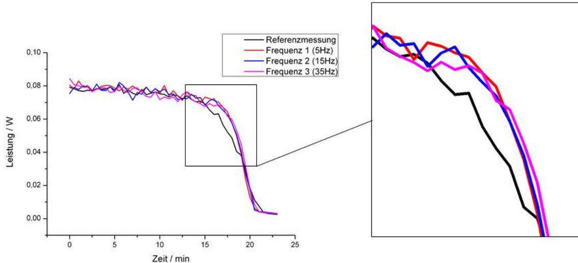
Abbildung 21: Referenzmessung und die gemittelten Messungen mit den verschiedenen Frequenzen
