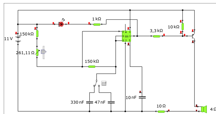
Abbildung 3: Schaltkreis des Rüttlers
