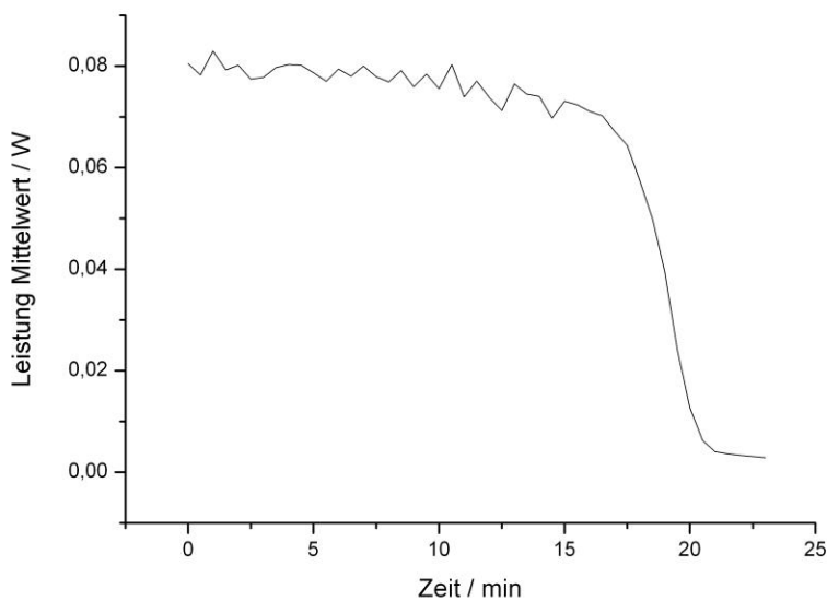
Abbildung 16: Gemittelte Messungen im Leistungs-Zeit Diagramm beim Rütteln mit 5Hz
