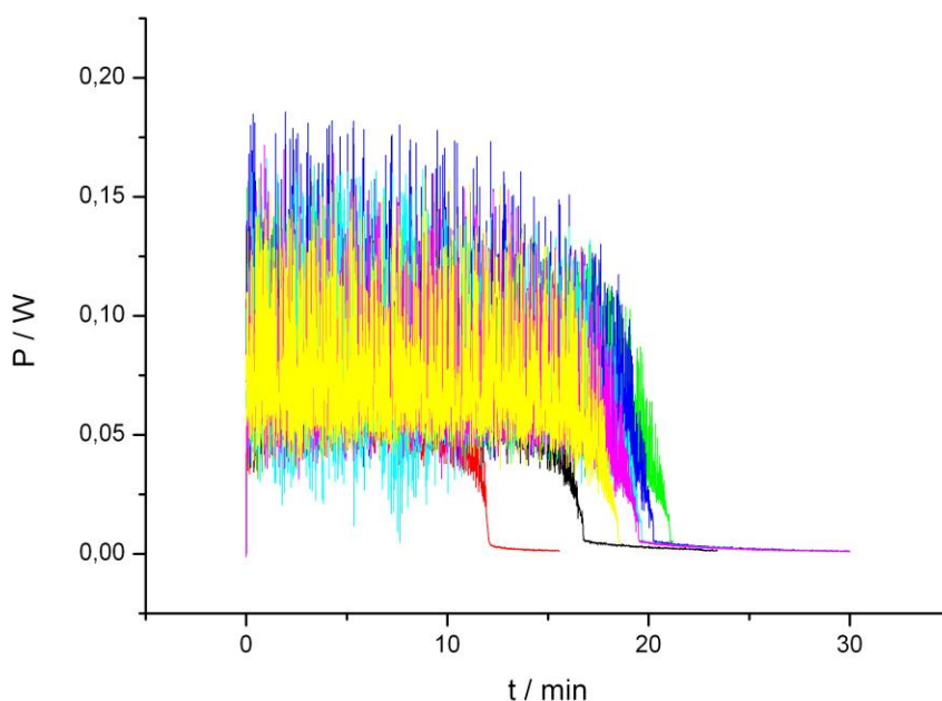
Abbildung 12: Sechs Messungen im Leistungs-Zeit Diagramm bei Normalbedingungen
